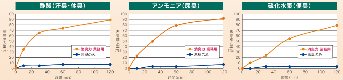
■消臭力 業務用 ビーズタイプ 消臭試験結果 (400g 無香料で実施) ※エステー調べ
